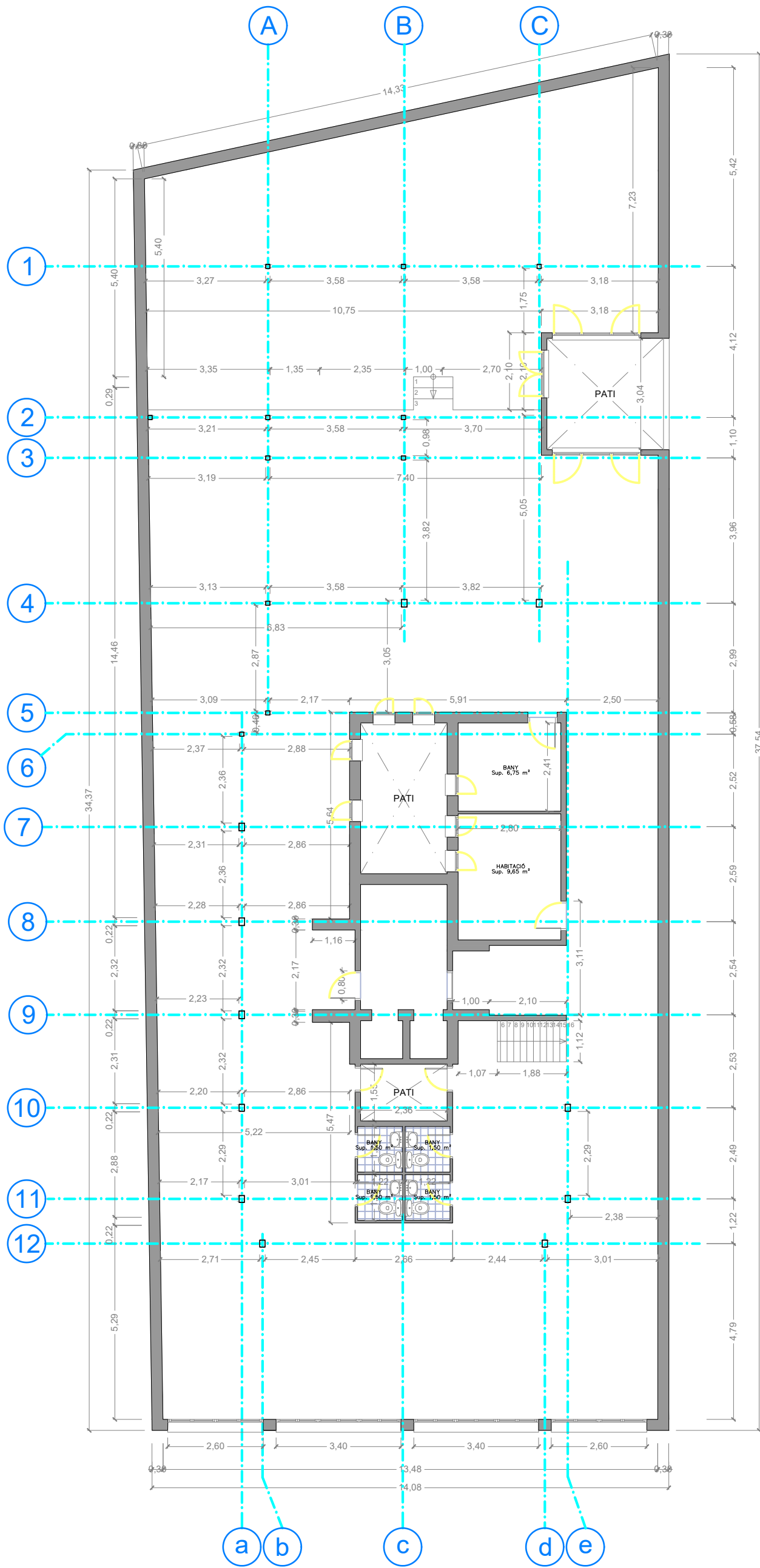
PLANTA ENTRESUELO Sup. construida 497,30 m2
